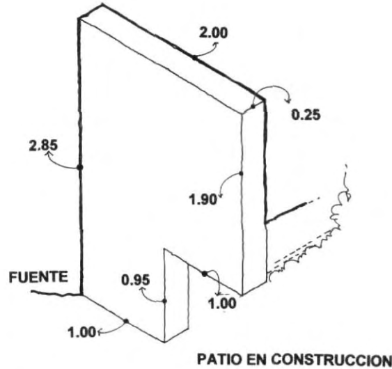
PERFIL DEL MURO
